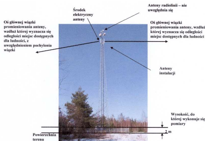
Rys. 32. Przykładowa instalacja radiokomunikacyjna wolnostojąca. Miejsca dostępne dla ludzi znajdują się na powierzchni terenu, za wyjątkiem wygradzonej i oznakowanej działki otaczającej instalację. Miejsca dostępne dla ludzi mogą znajdować się także pod osią główną wiązki promieniowania anteny.
