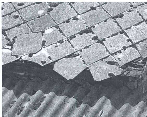
Rys. 8. Pokrycie dachowe ocenione w I stopniu pilności.
